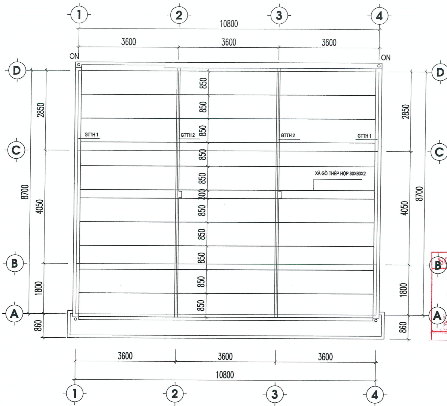
MẶT BẰNG XÀ GÒ MÁI
