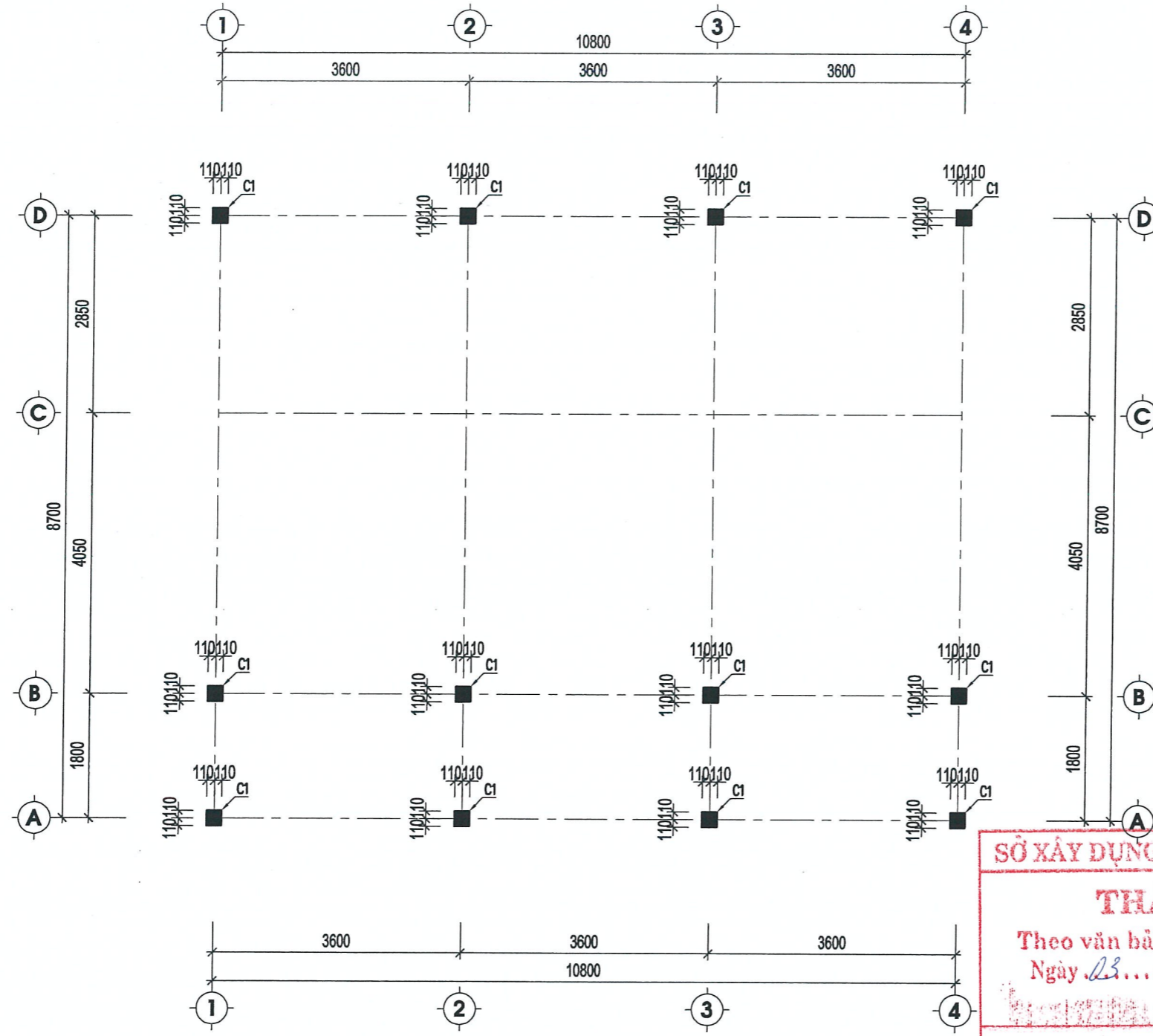
MẶT BẰNG ĐỊNH VỊ CỘT
