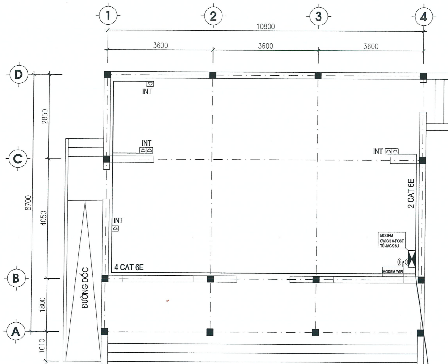
MẶT BẰNG LẮP ĐẶT MẠNG INTERNET
