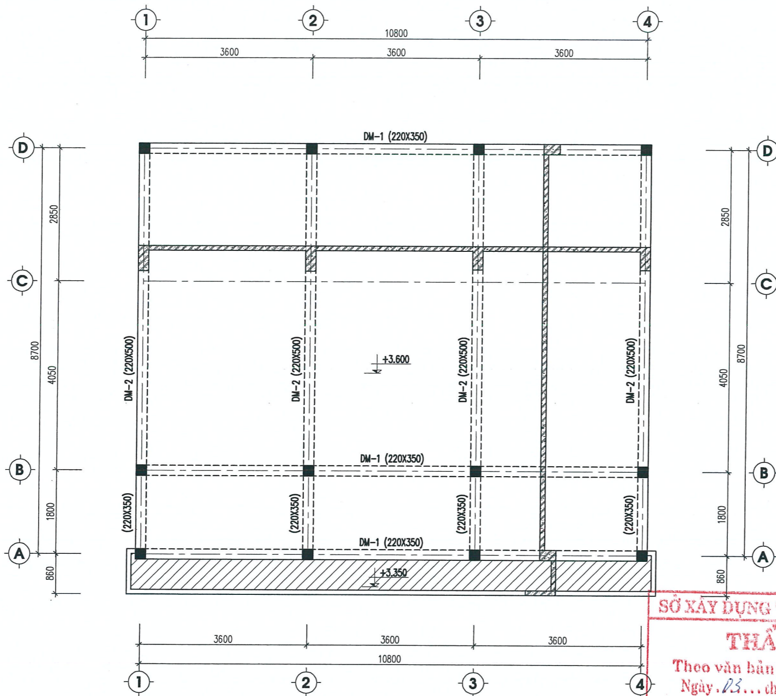
MẶT BẰNG KẾT CẤU MÁI
